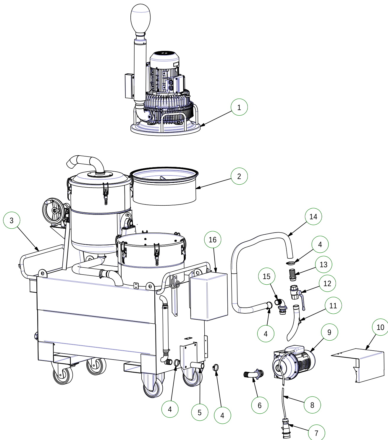
Part List / Elenco parti
